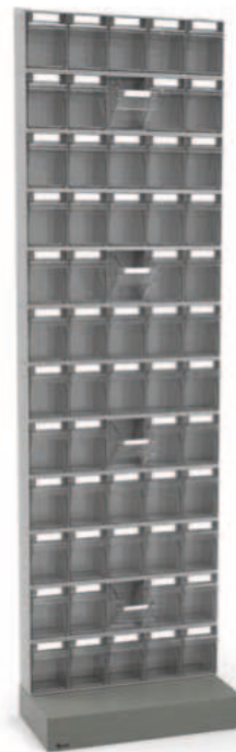
SCAFFALE CON 60 CASSETTI VISUAL BOX DIM. (mm): L=604 P=322 H=2100
